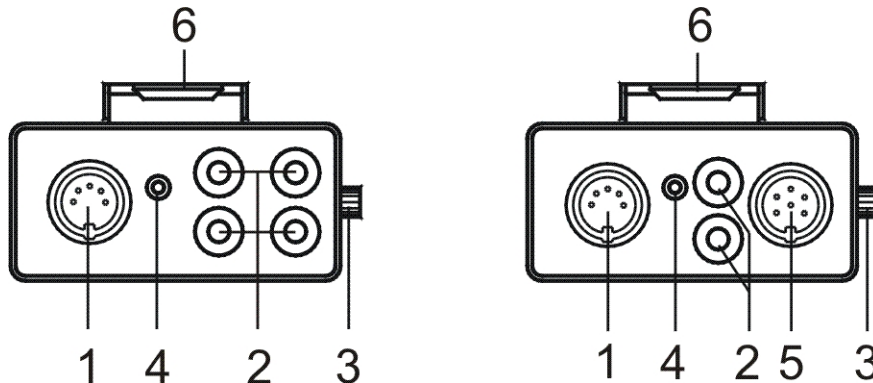
Sprechverstärker SV4-S mit Schalt-Taster
